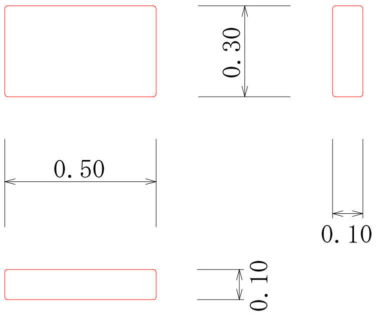
土のう仕上寸法
