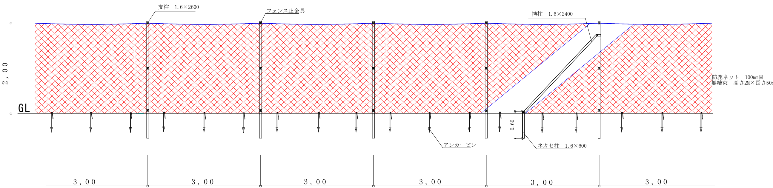
獣害防止ネット 材料表(支柱設置間隔3.0m) (100m当たり)
