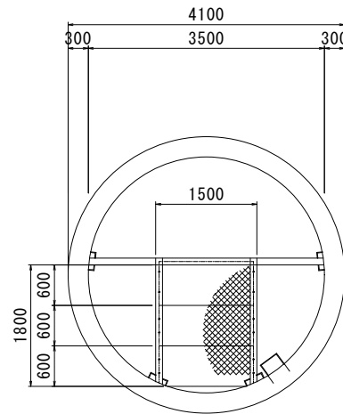
D-D平面図 S=1/50
