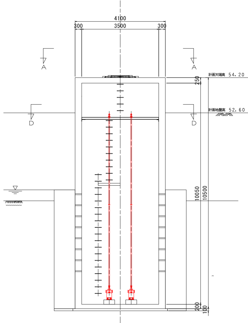
C-C断面図 S=1/50
