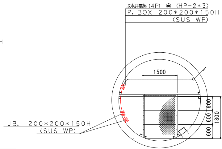
D-D平面図 S=1/50
