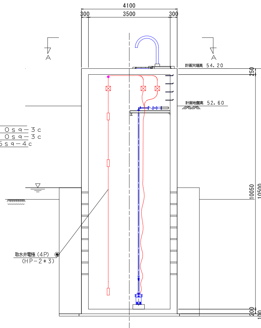
B-B断面図 S=1/50
