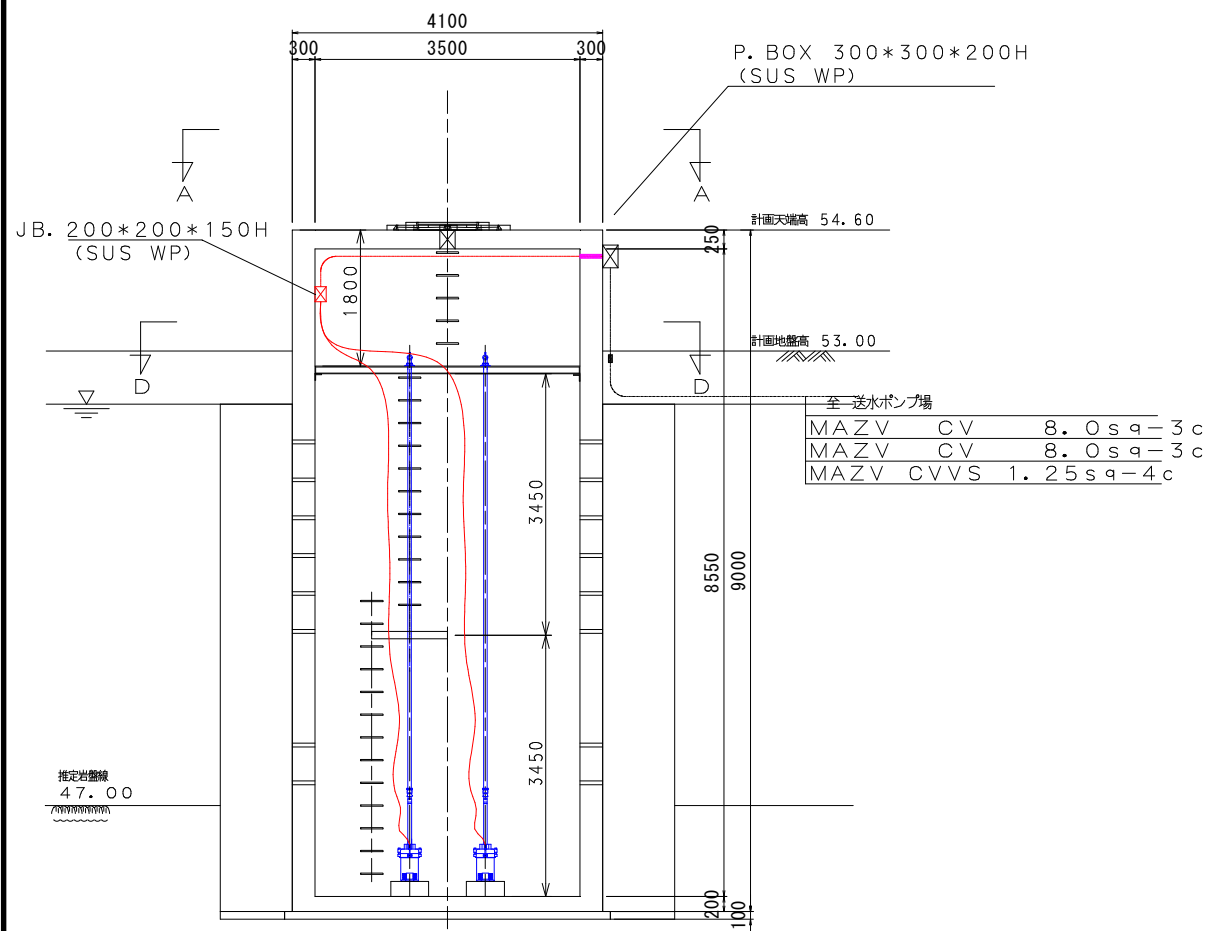
C-C断面図 S=1/50
