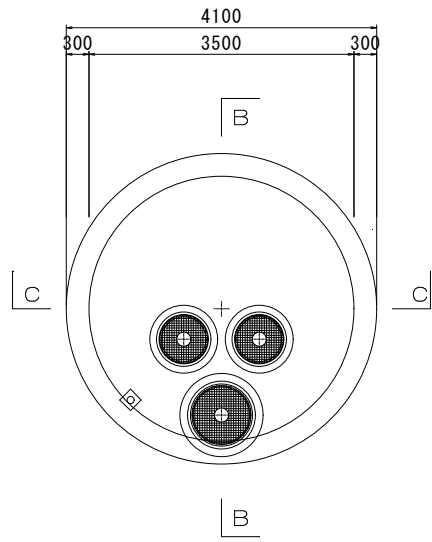
A-A平面図 S=1/50
