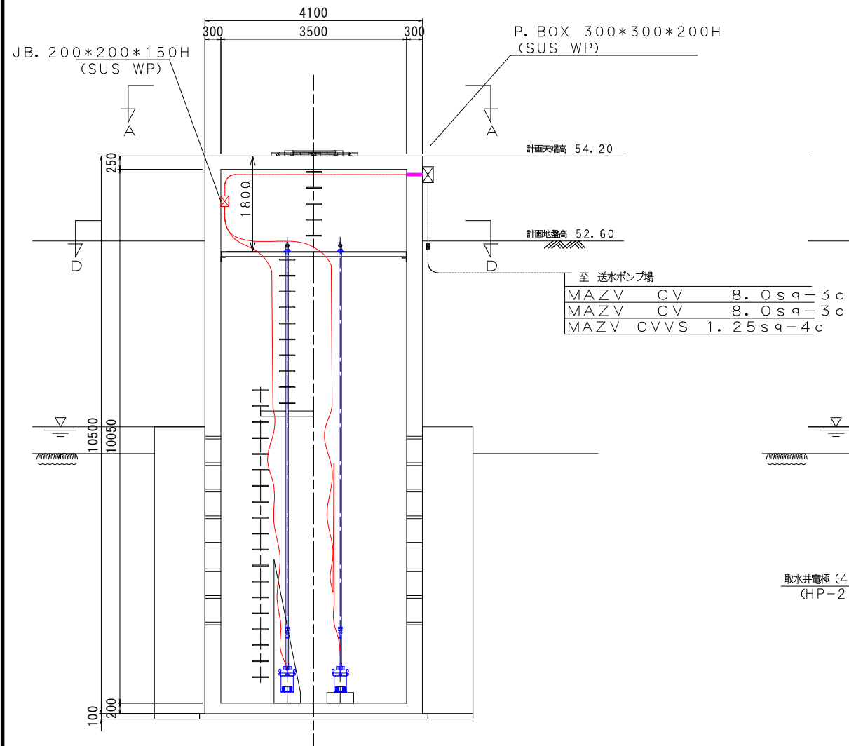
C-C断面図 S=1/50
