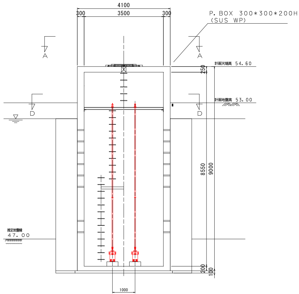
C-C断面図 S=1/50
