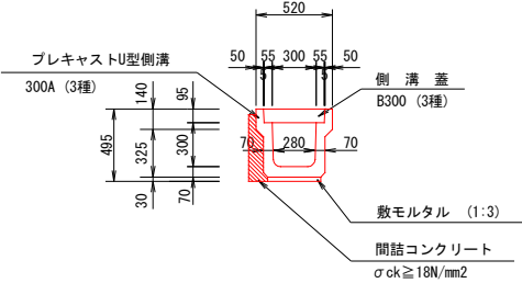
構 造 図 U型側溝 S=1:20
