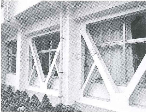
桜谷小学校 鉄骨ブレースにより補強
